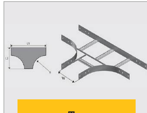
Tee
